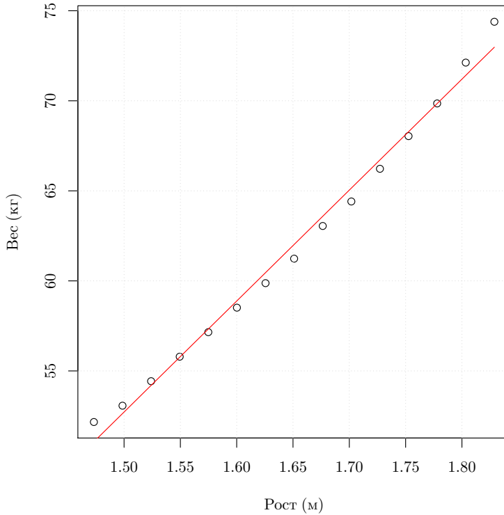
Рис. 22. Зависимость между ростом и весом
