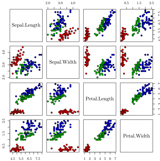
Рис. 33. Матричный график
