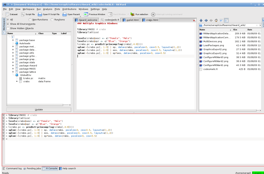
Рис. 67. Окно RKWard
