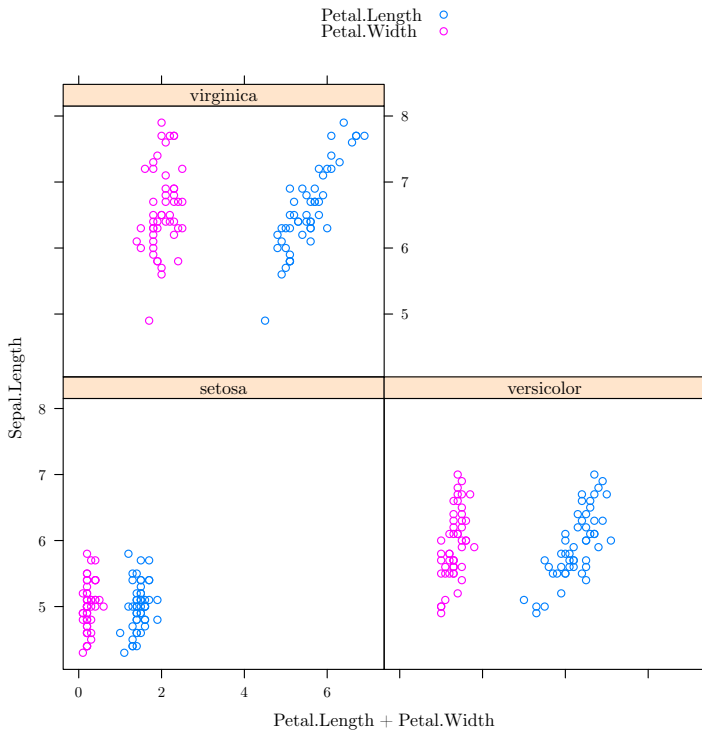
Рис. 31. Пример Trellis-графики
