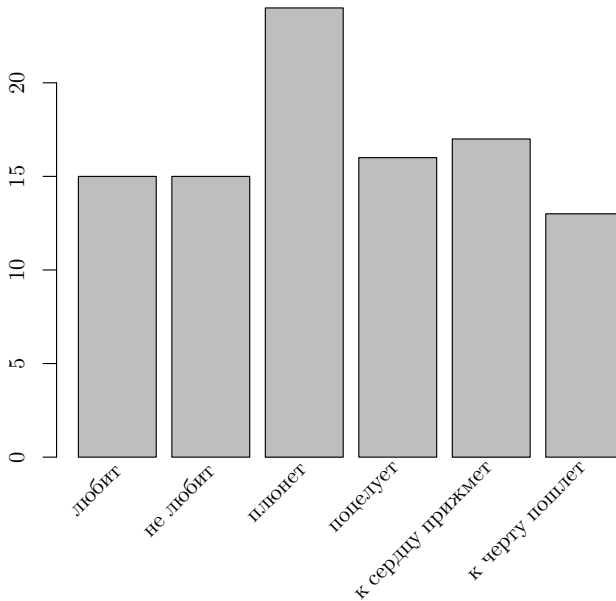
Рис. 7. Результаты гадания на ромашках (проценты исходов), показанные с помощью столбчатой диаграммы
