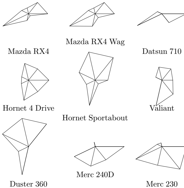
Рис. 34. Звезды изображают разные марки автомобилей
