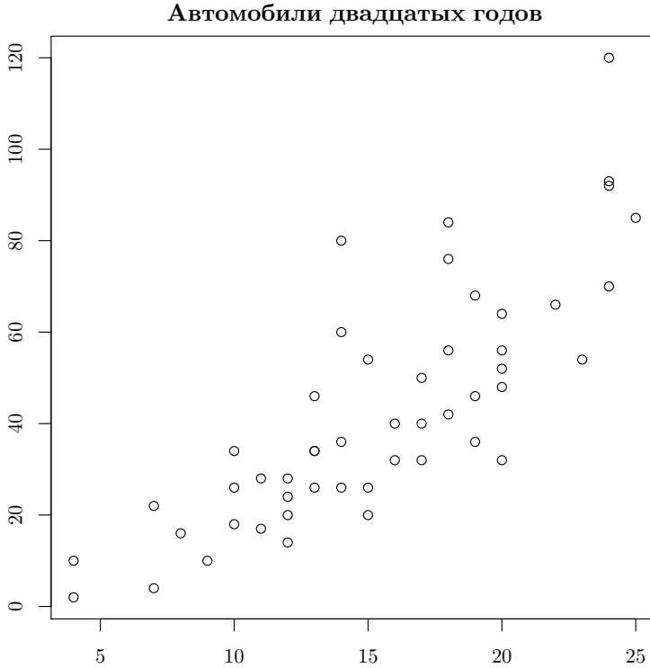
Рис. 2. Пример графика, отражающего встроенные данные cars
