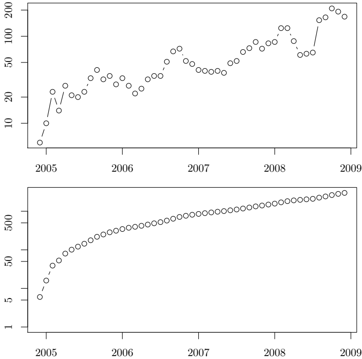
Рис. 57. Изменения месячного и общего количества пользователей
